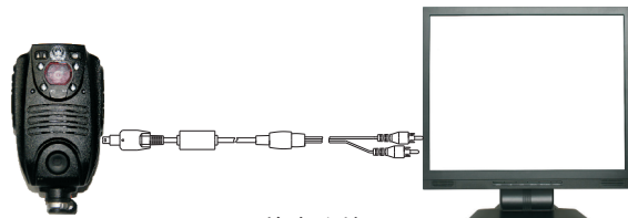
AV输出连接图
